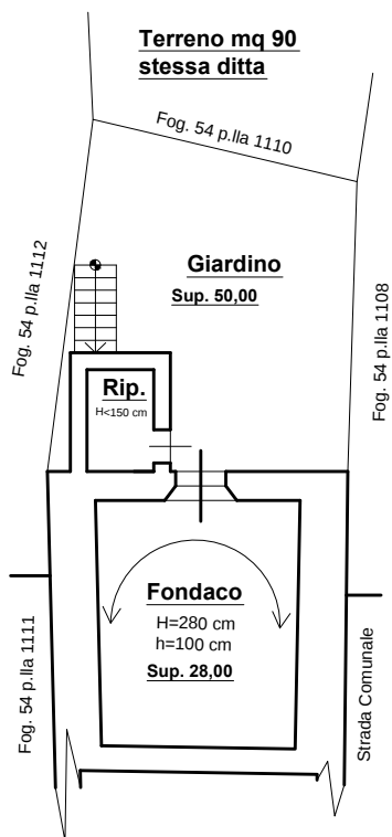
PIANTA PIANO SEMINTERRATO
